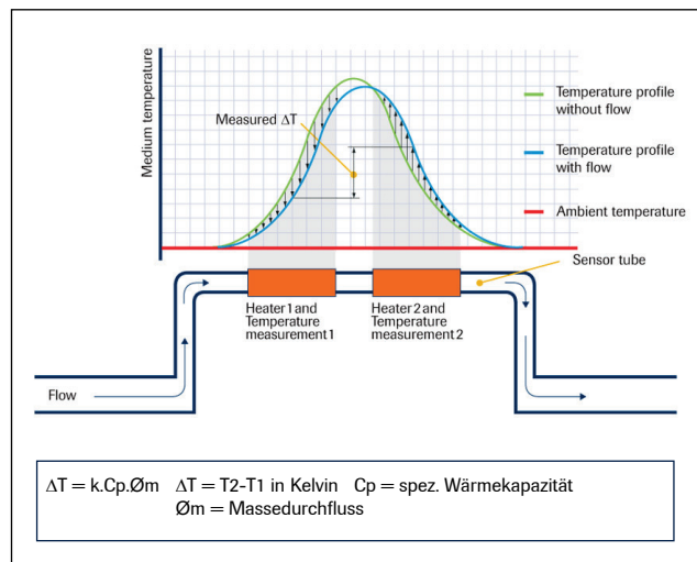
Funktionsschema thermischer Durchflusssensor F-110CI
